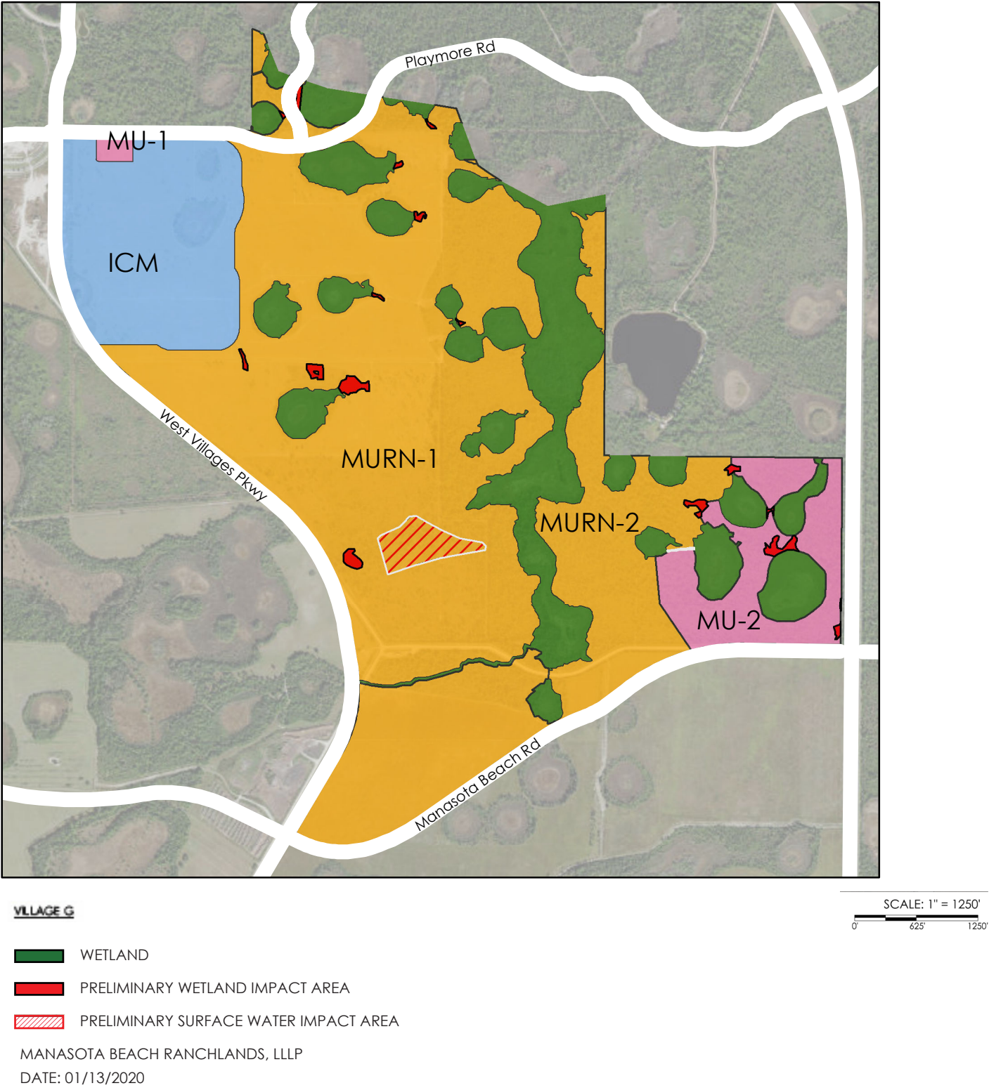
Figure 3.6.1.A Wetland Impact Plan
